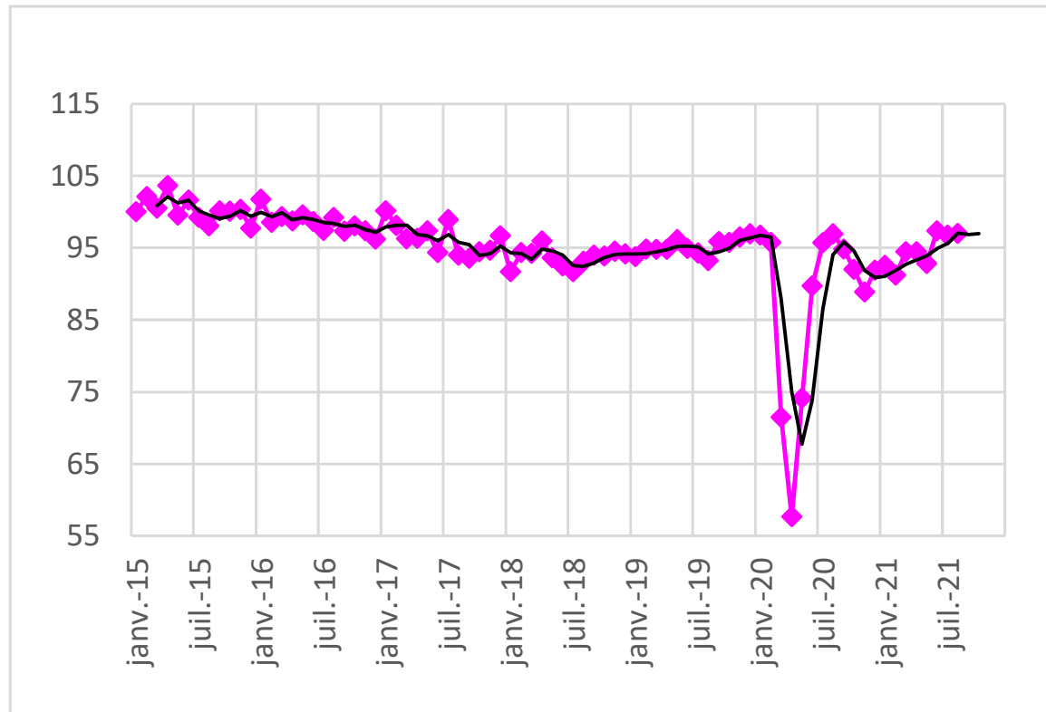
Evolution des remboursements mensuels CVS-CJO de cliniques en date de soins (base 100 = remboursements janvier 2015)
